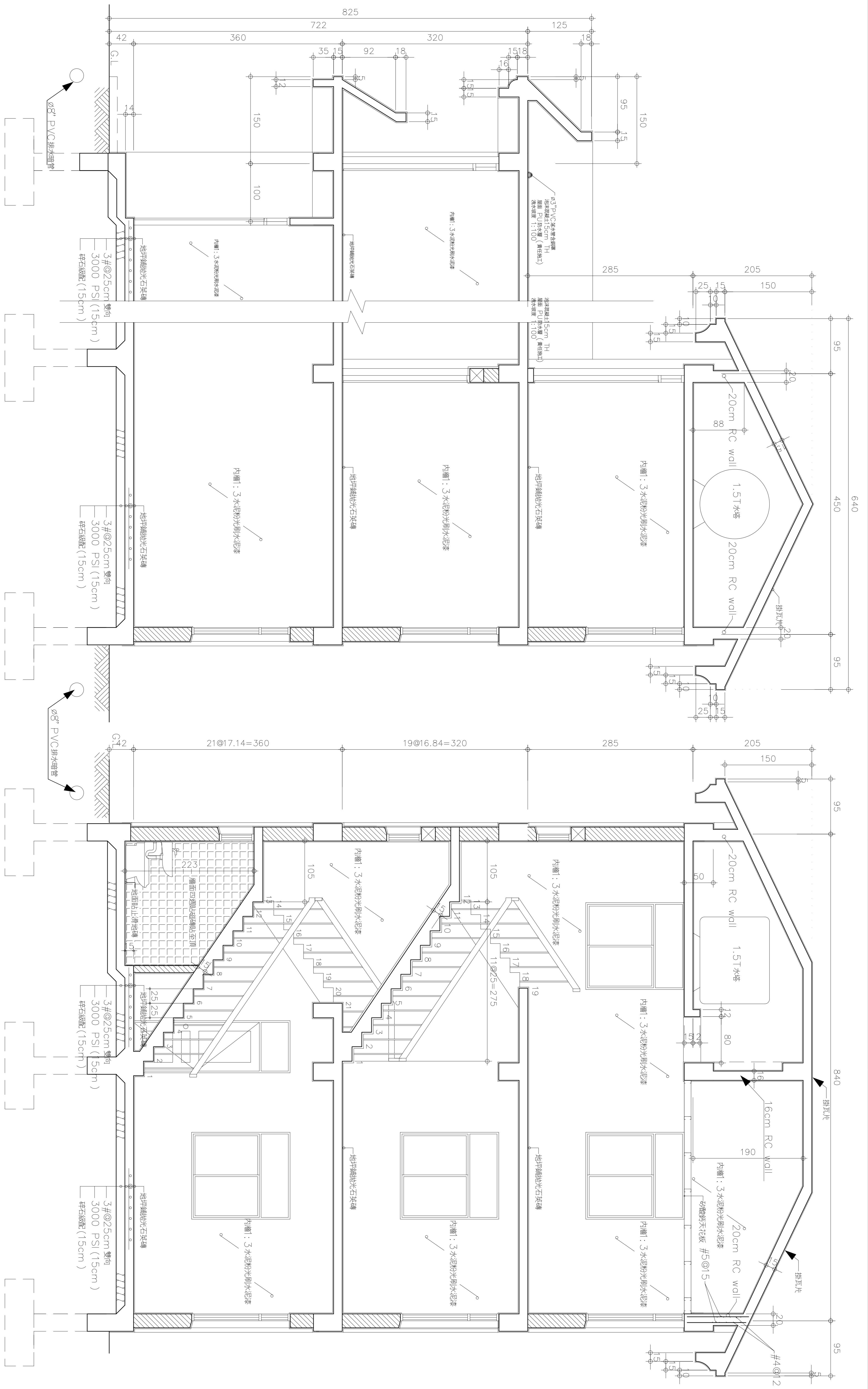
① 剖面詳圖 scale=1/20
